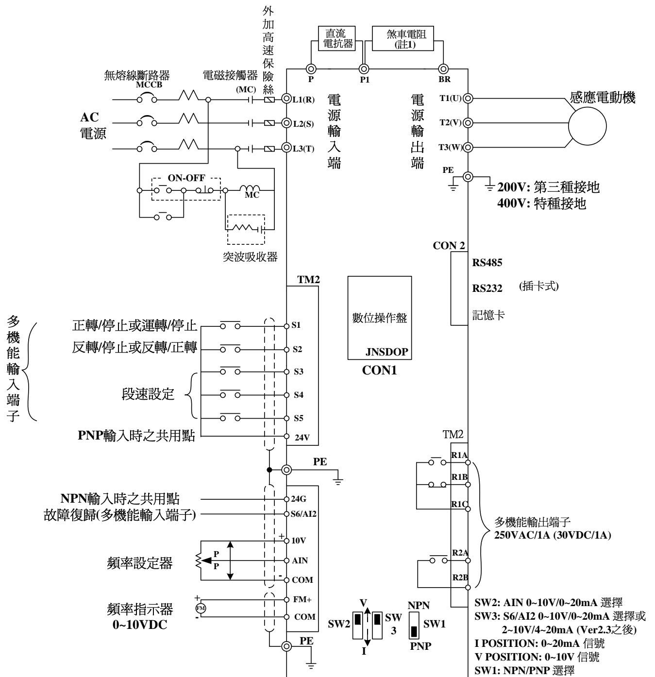
配線圖一
